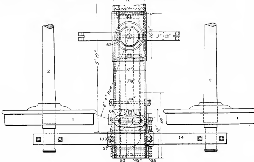
Fig. 4645. Part Plan.
